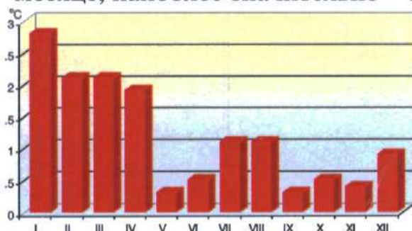
Рисунок 3.1.2 Отклонение среднемесячной температуры воздуха от среднемноголетних значений за 1989 – 2013годы
