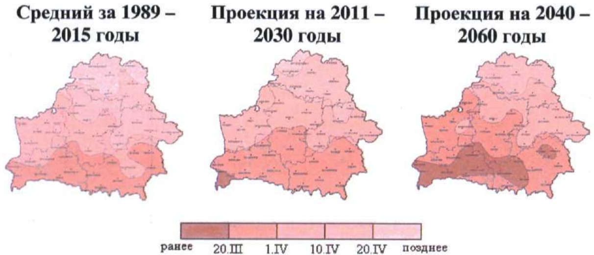
Рисунок 3.2.6 Срок наступления мягко пластичного состояния почвы (начало сева ранних яровых культур) для сценария RCP4.5
