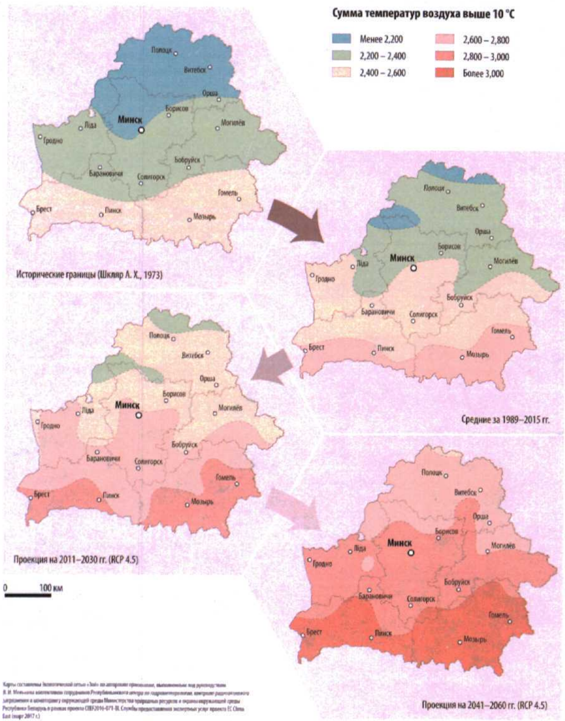
Рисунок 3.2.8 Историческое и ожидаемое для сценария RCP4.5 изменение границ агроклиматических зон Беларуси
