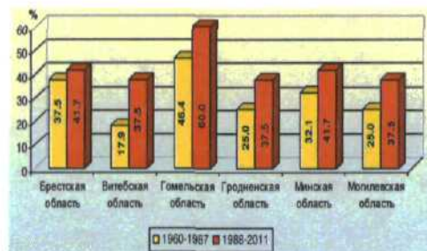
Рисунок 3.1.6 Повторяемость засух до и после потепления климата (2013 по данным Белгидромета)
