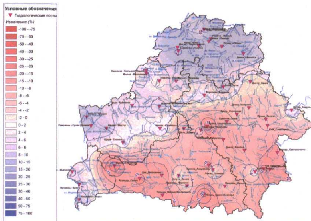
Рисунок 3.2.2 Прогноз изменения среднегодового стока к 2035 году (ЦНИИКИВР, 2016)
