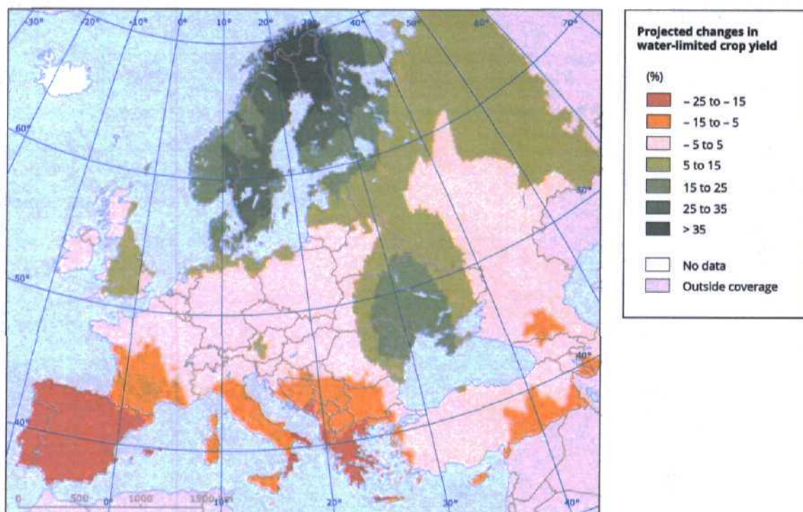
Рис 3.2.5 Среднее изменение (%) в Западной и Центральной Европе ограниченной влагозапасом урожайности пшеницы, кукурузы и сои в 2050 году по сравнению с 1961 – 1990 годами (EuropeanEnvironmentAgency, 2017 по даннымIglesiasetal., 2012, Ciscaretal., 2011)
