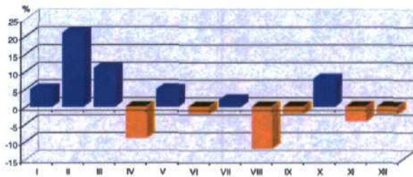
Рисунок 3.1.5 Отклонение (%) месячной суммы осадков за 1989 – 2013 годы от климатической нормы (2013 по данным Белгидромета)
