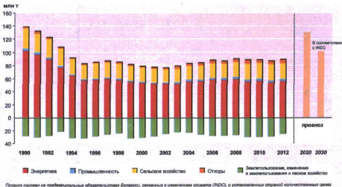
Рисунок 2.2.4 Выбросы парниковых газов в Беларуси и их ожидаемое изменение
