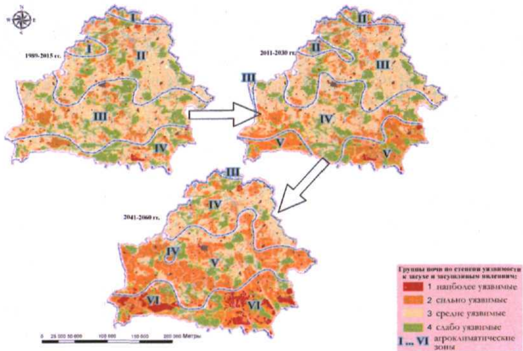
Рисунок 3.2.9 Современная и будущая (сценарий RCP4.5) уязвимость почв Беларуси к засухами засушливым явлениям
