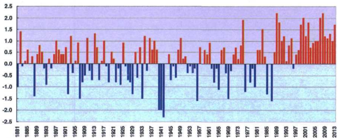
Рисунок 3.1.1 Отклонение средней по Беларуси среднегодовой температуры воздуха от климатической нормы (2013 по данным Белгидромета)
