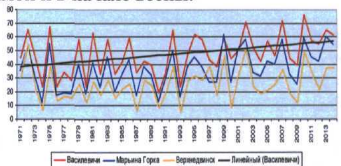
Рисунок 3.1.3 Число жарких дней (с максимальной температурой воздуха +25^{\circ}\text{C} и выше) в 1971 – 2013 годах (2013 по данным Белгидромета)
