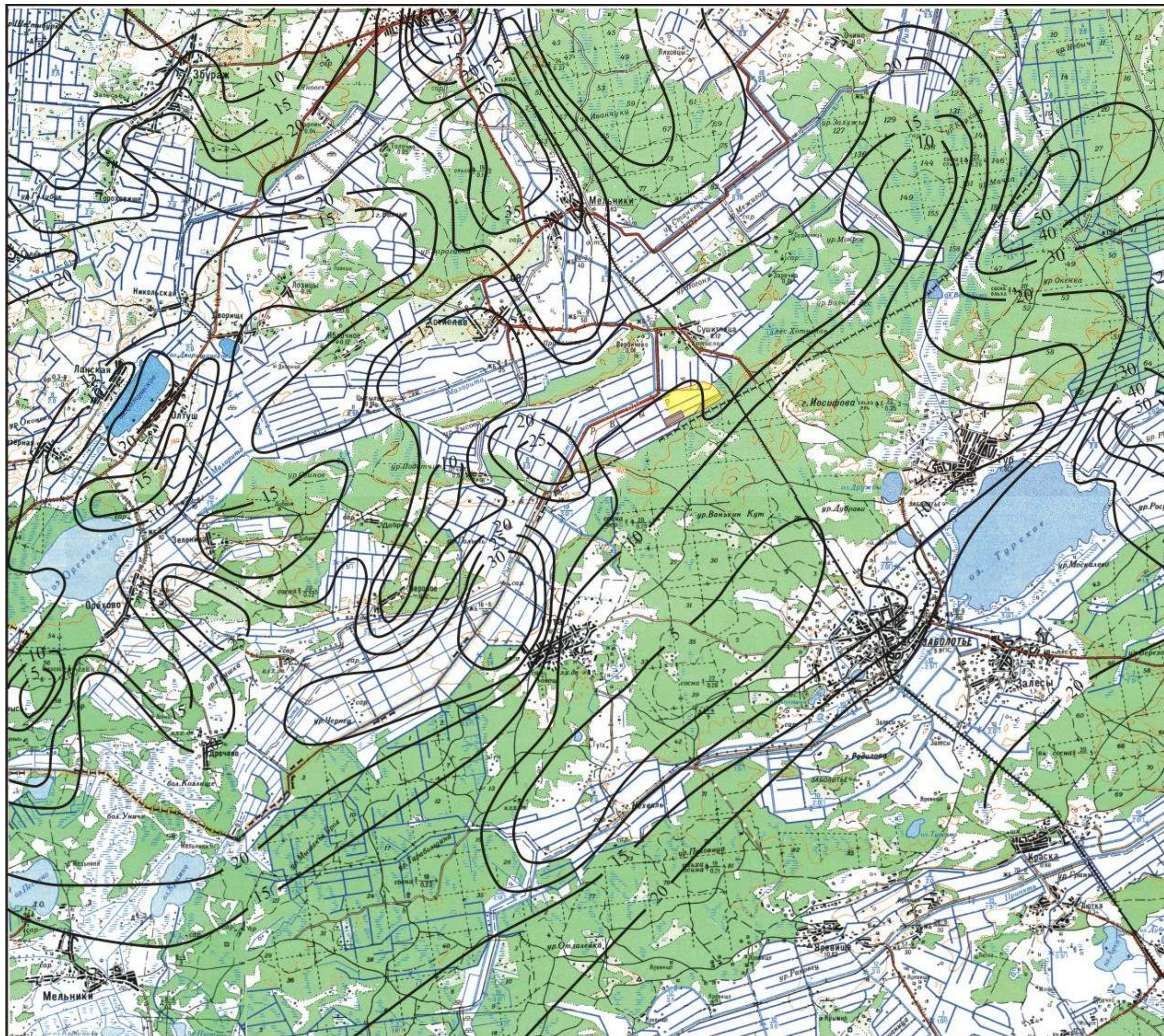
Карта-схема мощности водовмещающих отложений четвертичного водоносного комплекса. Масштаб 1:100 000
