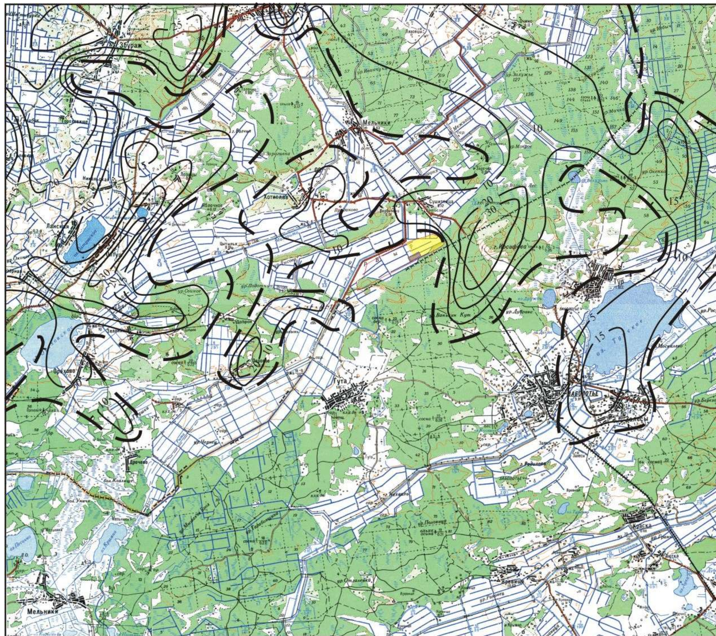
Карта-схема мощности слабопроницаемых четвертичных отложений. Масштаб 1:100 000
