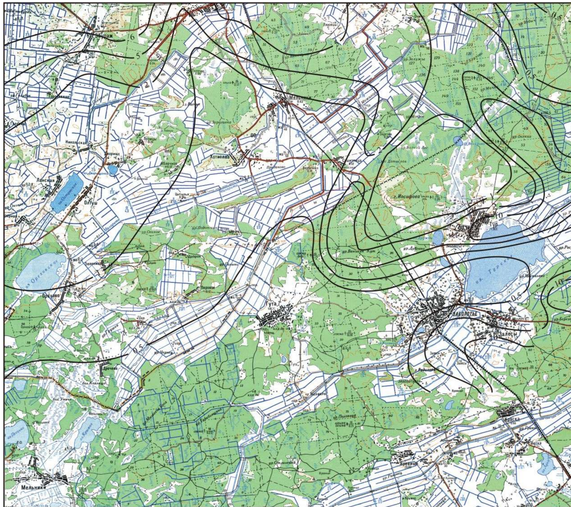
Карта-схема мощностей слабопроницаемых отложений зоны кольматации верхнего мела. Масштаб 1:100 000
