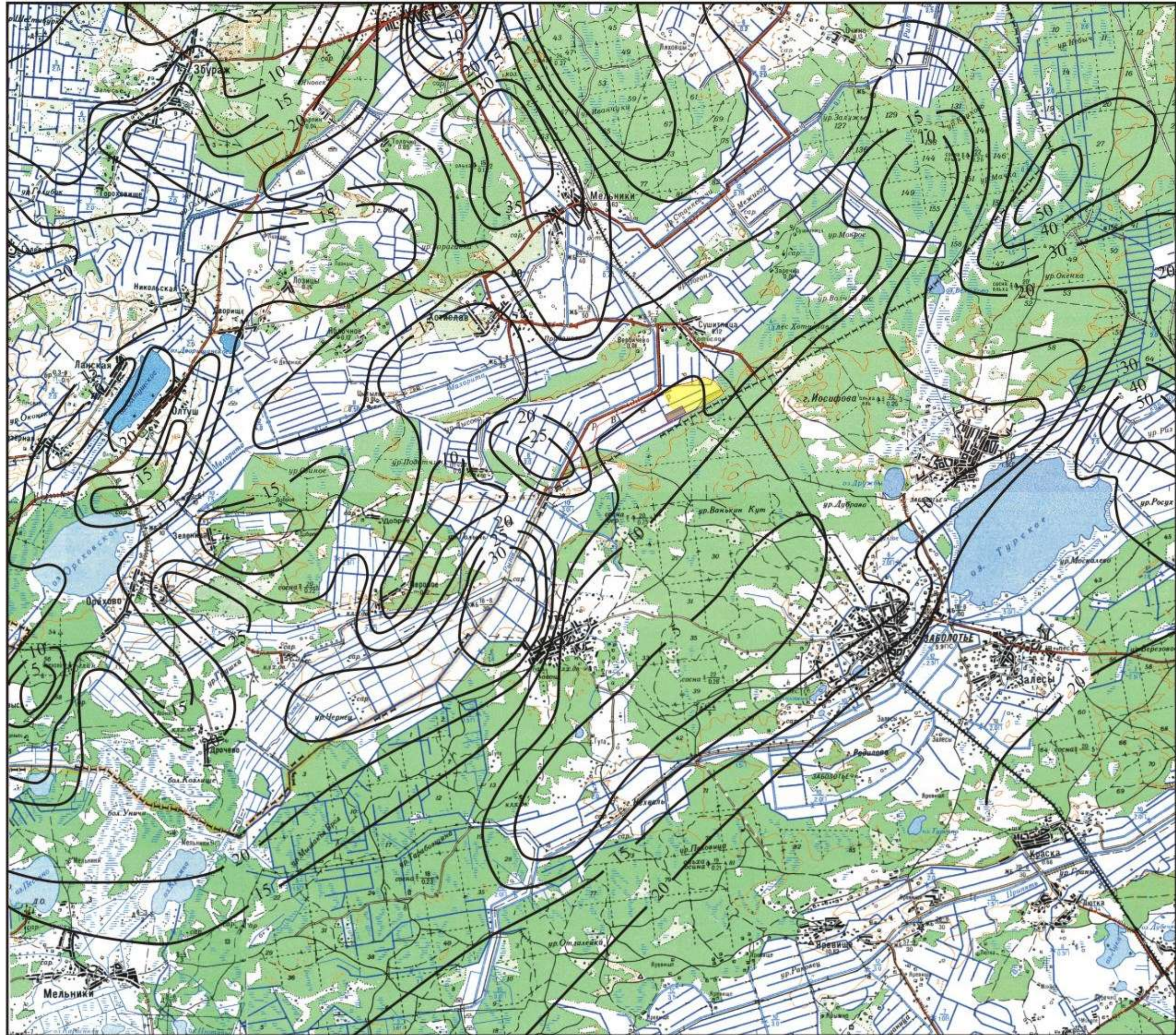
Карта-схема мощности водовмещающих отложений четвертичного водоносного комплекса. Масштаб 1:100 000
